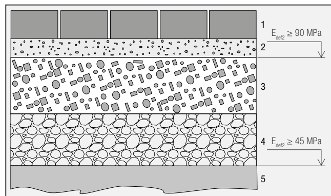
Skladba č. 3: Plocha s jezdem vozidel nad 3,5 t
