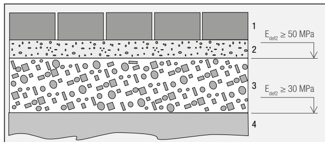
Skladba č. 1: Pochozí plocha
