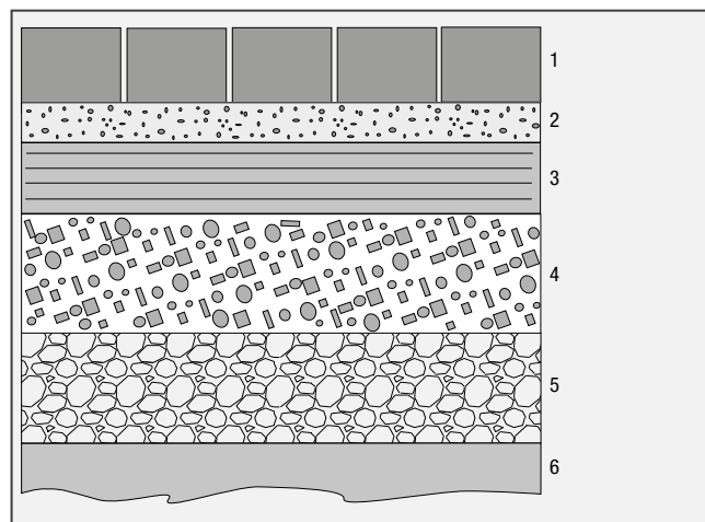
Skladba č. 4: Plocha s těžkým provozem
