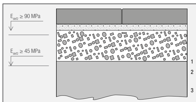
Skladba č. 1: Plochy s jezdem vozidel do 3,5 t (pro velkoformátovou dlažbu tl. 120 mm)
