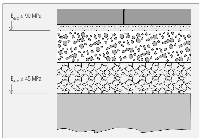
SKLADBA č. 2: Plochy s jezdem vozidel se zatížením max. 5t / kolo, resp. 10t / nápravu
