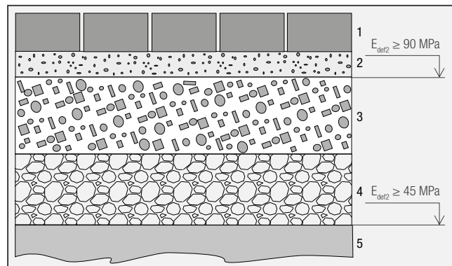
Skladba č. 2: Plocha s jezdem vozidel do 3,5 t
