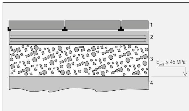
Skladba č. 2: Pochozí plochy – pokládka na vymešovaci terče
