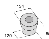
Spojovací kroužek RB-SK
