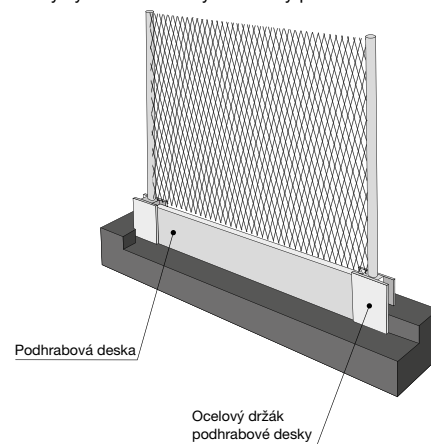
Plotová patka
