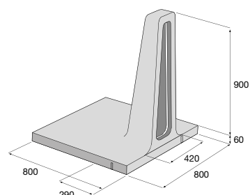
Dělicí sloupek G-ROW s osvětlením
