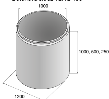
Betonová skruž TBX 2-100
