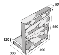
STANDARD S 55/R, reliéf – kámen
