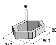
Vegetační dlažba H-E-X 80
