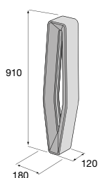
Dělicí sloupek H-E-X s osvětlením
