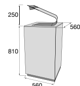
Koš TAMPA s oklepávkem str. 145
