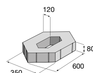
Vegetační dlažba H-E-X 120
