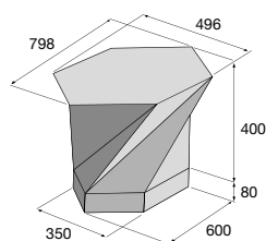
Sedák H-E-X DEFORM
