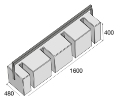
Stojan na kolo BLOCK str. 145
