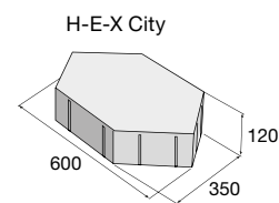
H-E-X City – podélná půlka
