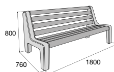
Lavička MARKO str. 136
