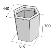
Koš SEISAVO str. 145
