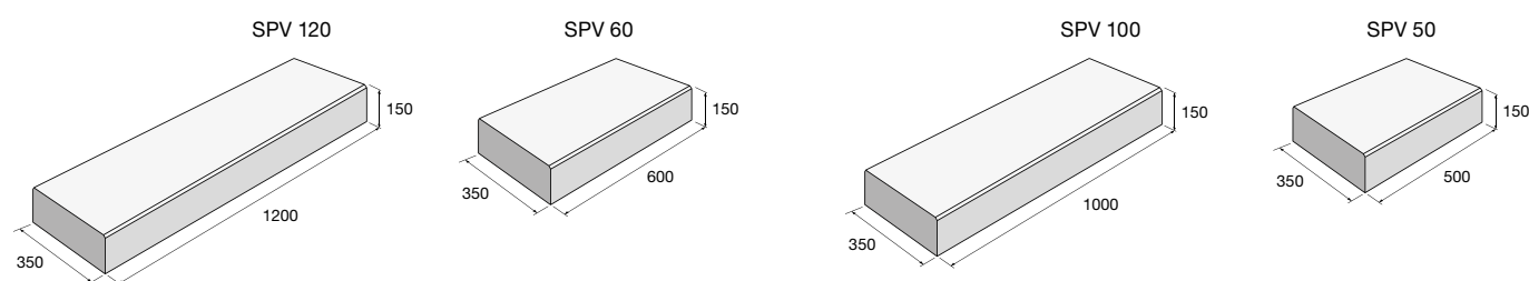
Stupeň přímý SPV – přírodní
