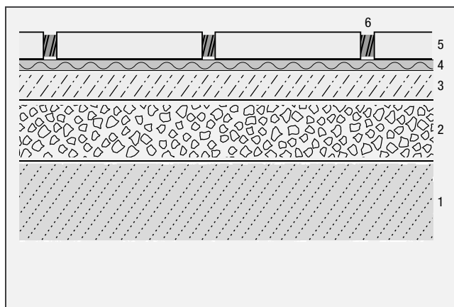
Skladba č. 7: Betonová plošná dlažba nalepená na stávající betonovou desku (ochoz bazénu, terasy na rostlém terénu, pochozí plochy popř. pojízdné se zatížením do 3,5 t) – [pěší] – [vozidlo]
