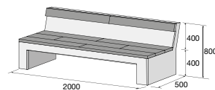
LAGUNA s opěradlem str. 136
