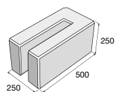
Stojan na kolo BLOCK MINI str. 145
