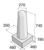
Dělicí prvek DELTA str. 146
