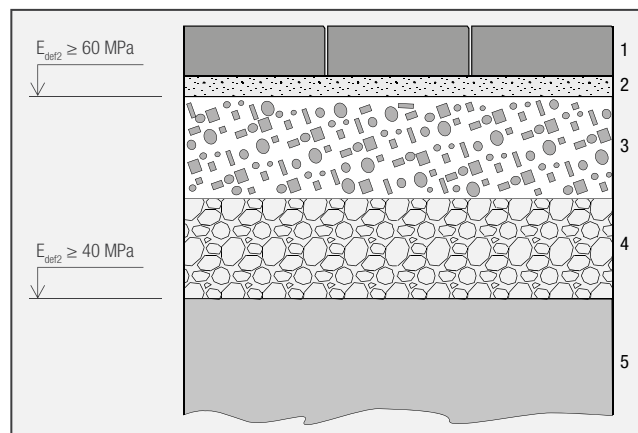
Skladba č. 8: Plochy s občasným jezdem do 3,5 t (pro dlažbu tloušťky 62 mm) – [vozidlo]
