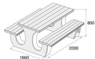
Piknikový stůl str. 142
