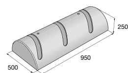
Stojan na kolo SK 2-3 str. 145
