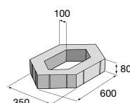
Vegetační dlažba H-E-X 100
