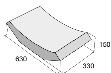
Příkopový žlab
