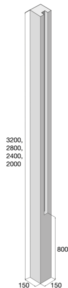
Sloupek koncový, reliéf – kámen
