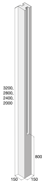
Sloupek průběžný, reliéf – kámen
