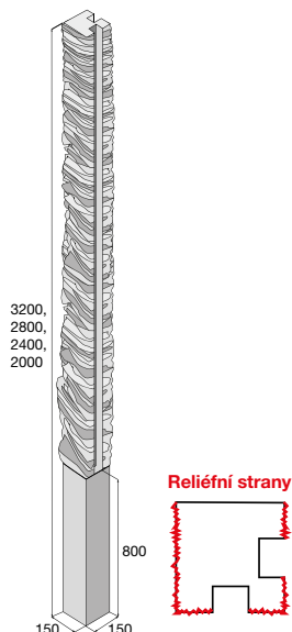
Sloupek rohový, reliéf – kámen
