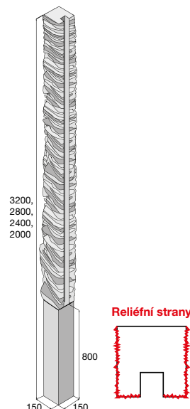
Sloupek koncový, reliéf – kámen
