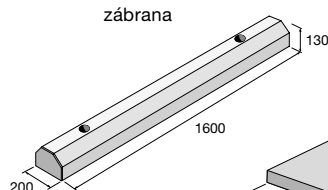
Parkovací zábrana
