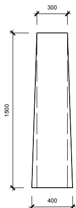
Půdorys
