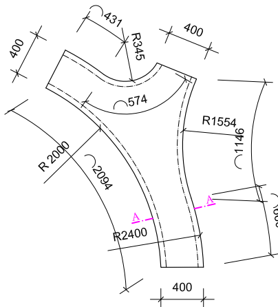
Půdorys
